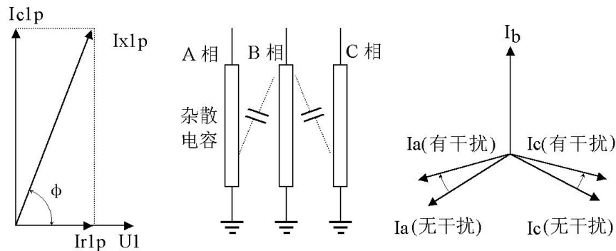
图 8 投影法 图 9、一字排列避雷器的相间干扰
