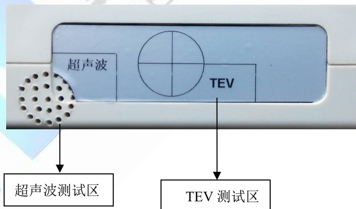
主机顶端图
