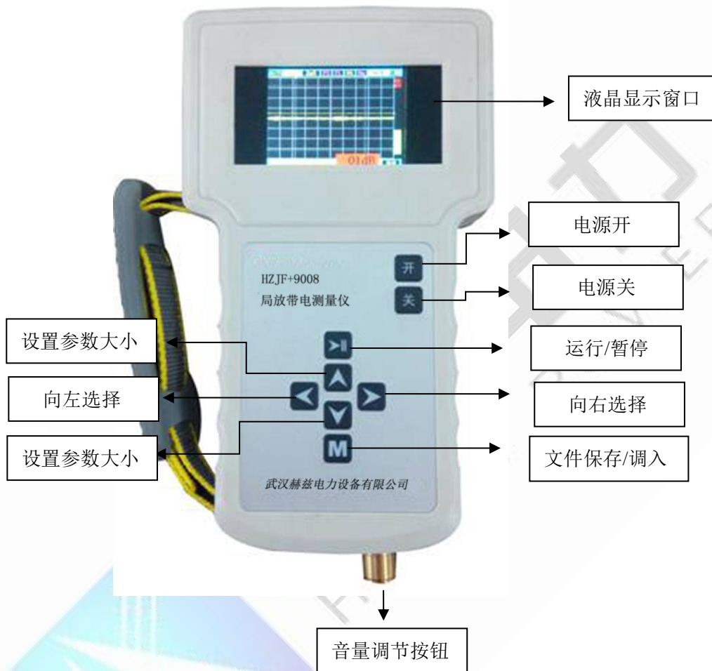
主机正面图
