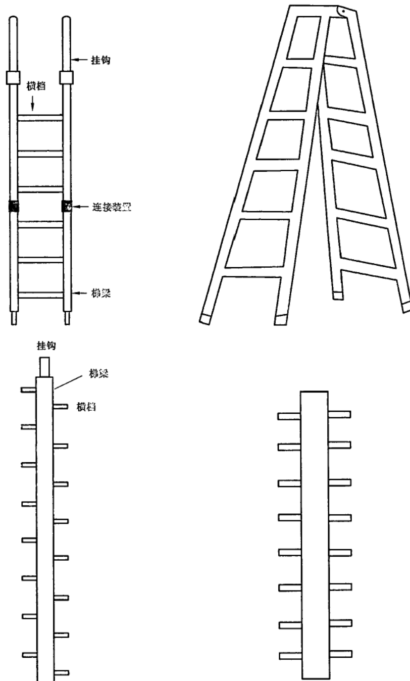
图 A.1 绝缘梯示意图
