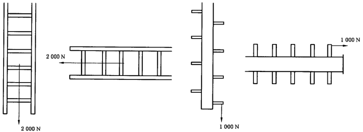
图 B.2 横档强度试验布置图
