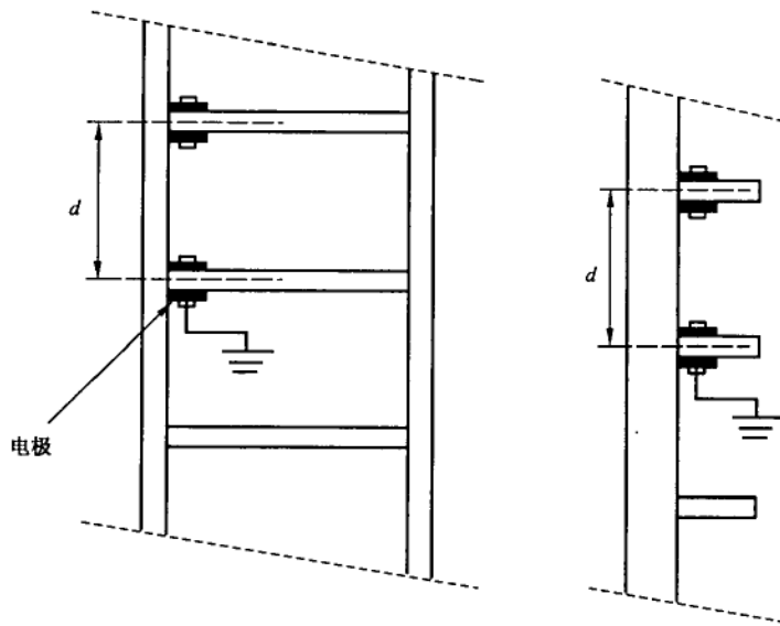
图 B.12 机械老化后电气试验布置图
