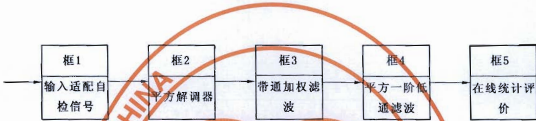
图 A.1 IEC 闪变仪模型的简化框图
