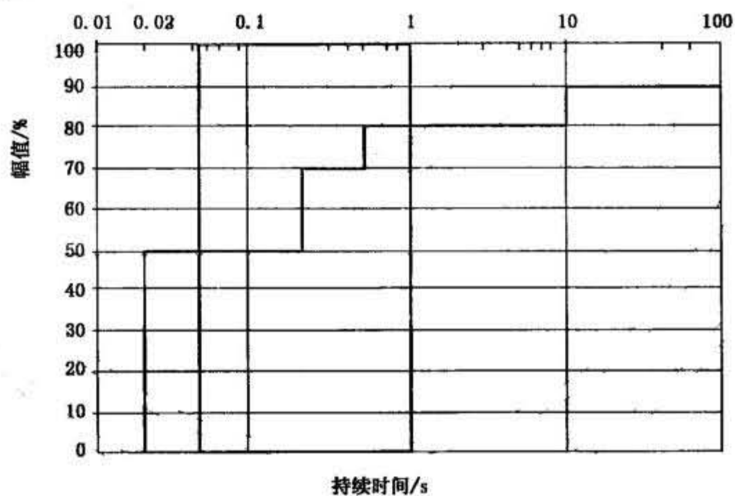
图 A.3 SEMI F47 曲线
